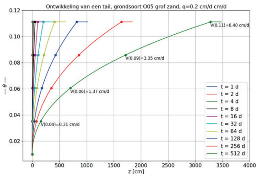
Afbeelding 6 Groei van de staart na plotselinge daling van de toevoer van 0.2 cm/d naar 0, waardoor het vochtgehalte op z=0 plotseling daalde van 12% naar veldcapaciteit. Elk puntje van deze staart heeft de snelheid die hoort bij zijn vochtgehalte. De puntjes behouden hun vochtgehalte en de daarbij behorende snelheid, zodat de staart lineair in de tijd naar rechts (naar beneden dus) wordt opgerekt, geheel onafhankelijk van wat zich verder boven- of benedenstrooms afspeelt.
