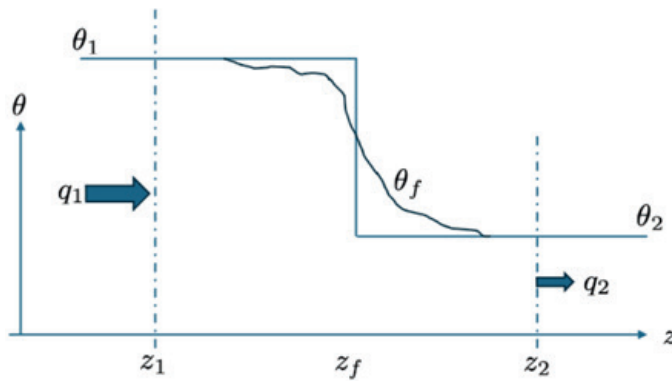
Afbeelding 9 Progressie van een vochtfront
